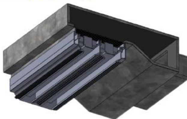
КСД-У торцевой врезкой
