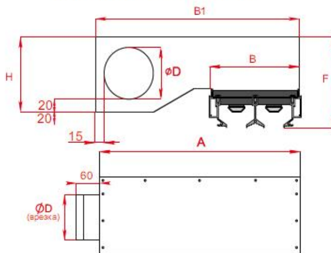
КСД-У торцевой врезкой
