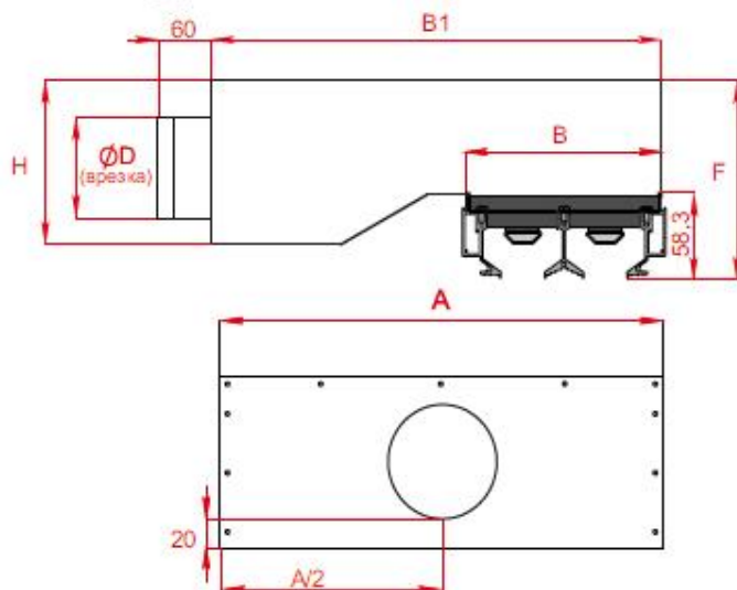
КСД-У с боковой врезкой
